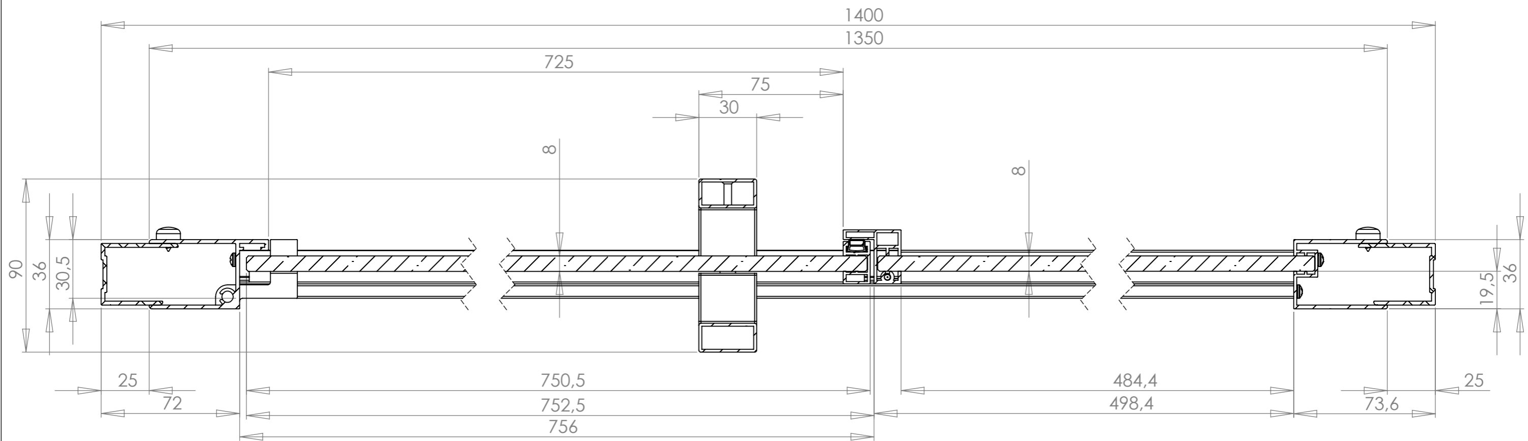
SECTION D-D SCALE 1 : 2
