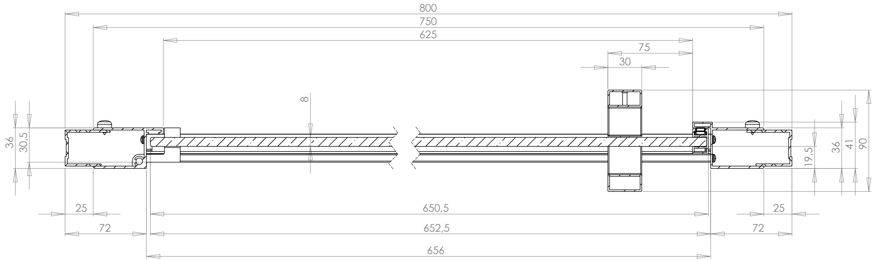
SECTION A-A SCALE 1 : 2
