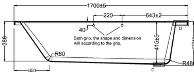
A-A
