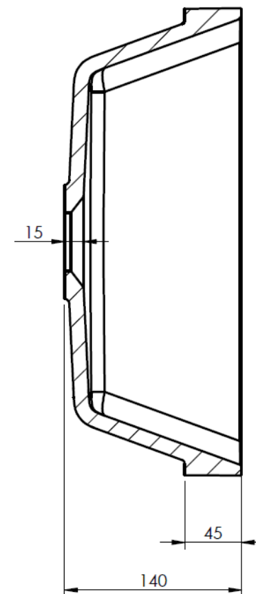
SEZIONE D-D
