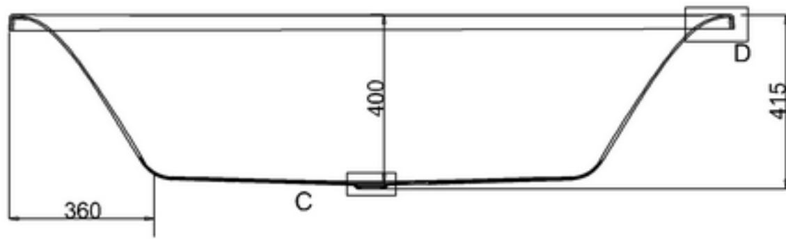
A-A
