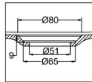
C SCALE 1:2
