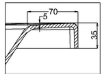
D SCALE 1:2
